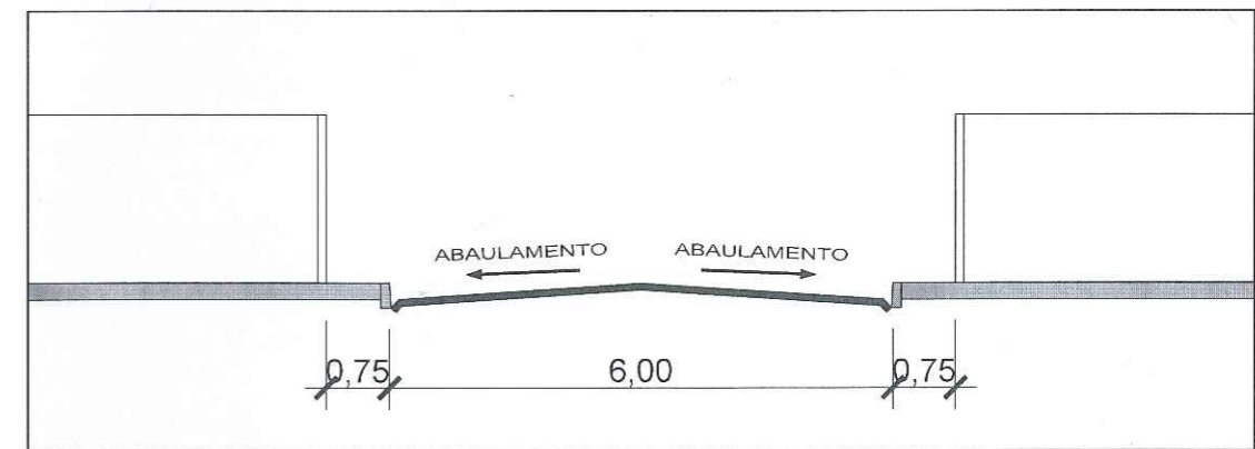
SEÇÃO TRANSVERSAL DA VIA - RUA ROQUE CALAGE Esc: 1/100
